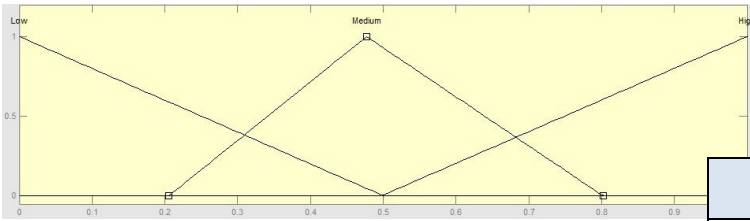
Fig.3. Fuzzy sets for semantic parameter
